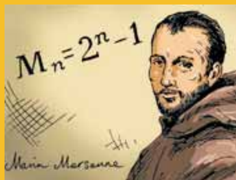
Θεώρημα Zsigmondy
